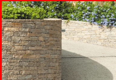
Pour stabiliser les aires, un mur de soutènement a été construit sur les trois quarts du tracé. Des traversées de route, avec grille en fonte, ont été aménagées tous les 10 m.
