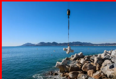
Numéroté et pesé, chaque bloc est placé sur la digue selon un plan de calepinage très précis réalisé en 3D.
