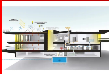
Coupe environnementale.
