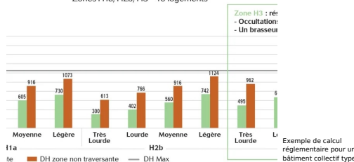
Fig. 5 Influence de l'inertie sur l'inconfort estival DH Zones H1a, H2b, H3 - 40 logements
