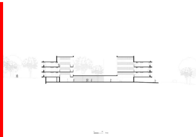
Coupe sur le hall transversal
