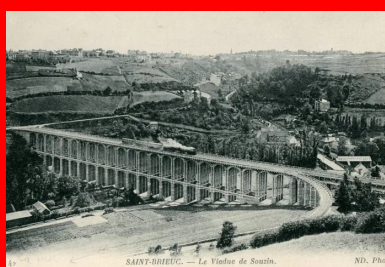
Construit à Saint-Brieuc en 1904, le viaduc de Souzain était un ouvrage complexe en trois parties : un ouvrage principal et une dérivation. D'une longueur totale de 274 m pour une hauteur de 35 m et une largeur de 11,40 m, il a été détruit le 27 juin 1995. (© DR)
